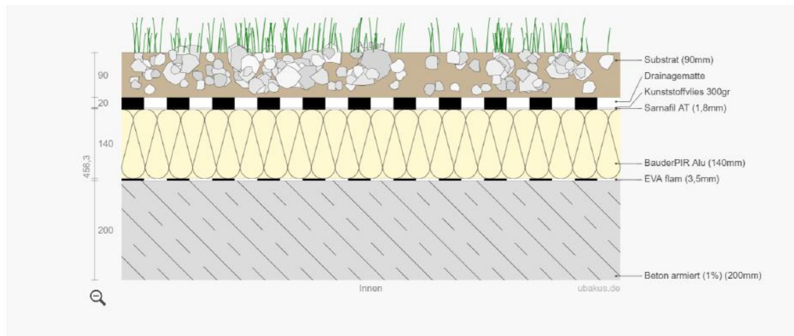
Abbildung 4: Neuer Aufbau
